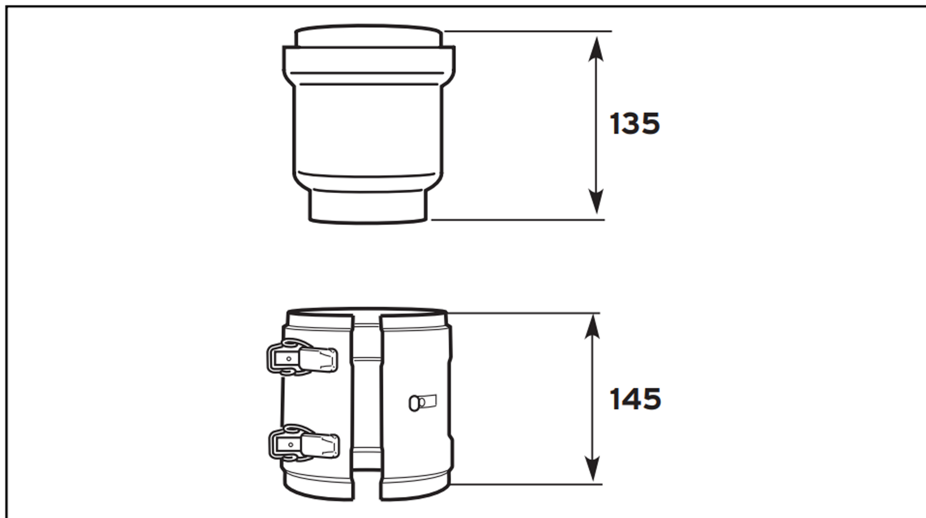
Fig. 4.7 Separatore, Ø 60/100
