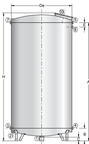
PASSO D'UOMO DECENTRATO PER MODELLI DA 3000 A 15000
