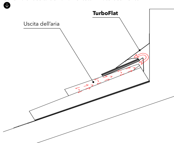
Schema di uscita dell'aria nei tetti in laterocemento
