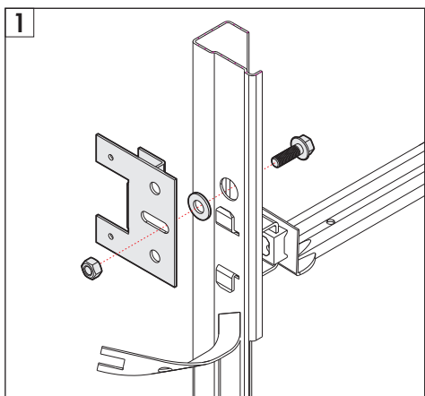
Fig. 1 Montaggio delle 8 staffe metalliche (4 per lato): è necessario interporre la rondella tra staffa e controtelaio.
