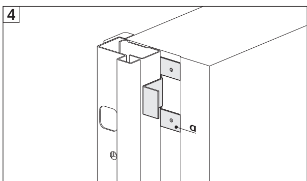
Fig. 4 Il montaggio delle parti in legno parte da una situazione di controtelaio e telaio già montati e fissati. Il controtelaio deve essere predisposto per il kit imbotte, ovvero con le apposite staffe (a) già montate.
