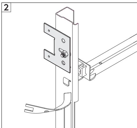
Fig. 2 Particolare montato
