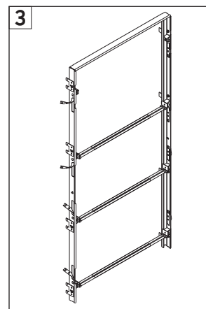
Fig. 3 Controtelaio finito
