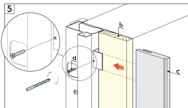
Fig. 5 Montare il supporto in legno (b) delle dimensioni adeguate sulla parete. Incastrare l'elemento del kit imbotte dotato dell'apposita fresata (c) sulle staffe e fissare il tutto con viti autofilettanti (d) , dopo avere pre-forato con un trapano.
