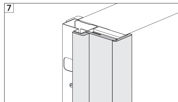
Fig. 7 Kit imbotte montato. N.B. è consigliabile usare collanti di tipo siliconico per il fissaggio degli elementi.
