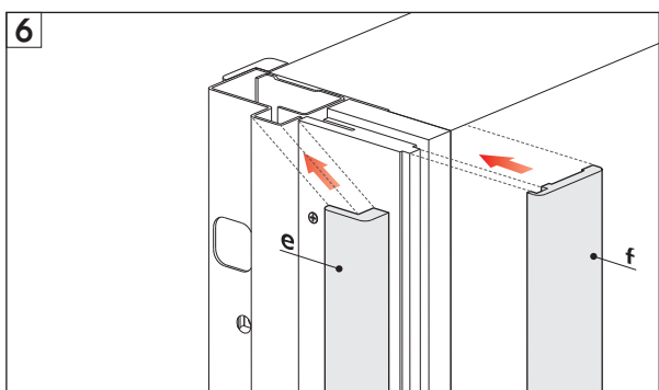
Fig. 6 Montare l'angolare copritelaio (e) ed infine il coprifilo del kit imbotte (f) incastrandolo sull'elemento montato precedentemente (c) .
