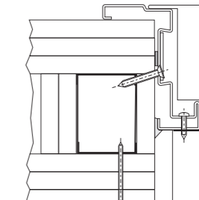
MONTAGGIO SU PARETE IN CARTONGESSO E l 120 E l 120 PLASTERBOARD WALL MOUNT
