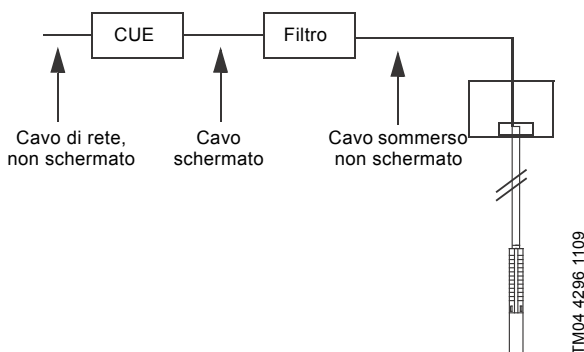
Fig. 23 Esempio di installazione in ambienti non sensibili all'EMC
