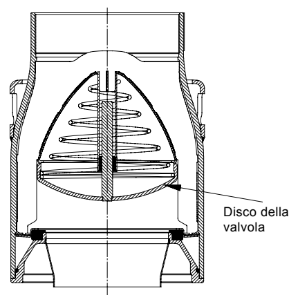
Fig. 5 Valvola di non ritorno
