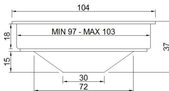
VISTA FRONTALE
