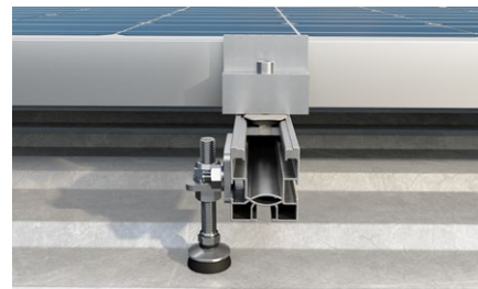
Copertura con rivestimento in lamiera grecata
